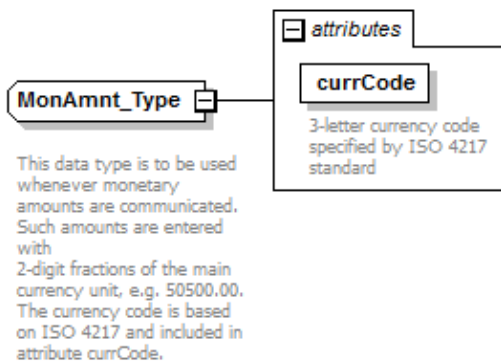
Figure 2 - MonAmnt_Type element
